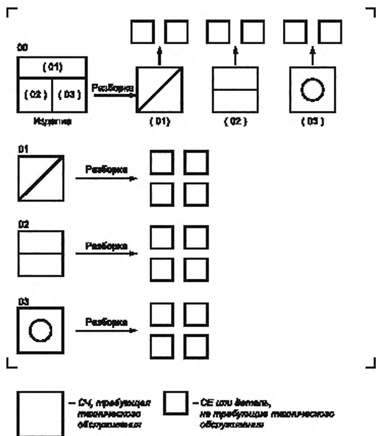
Рисунок Е.3 — Применение порядка разборки для нумерации S4
